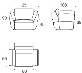
poltrona armchair
