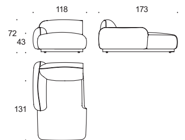
chaise longue sx lh chaise longue
