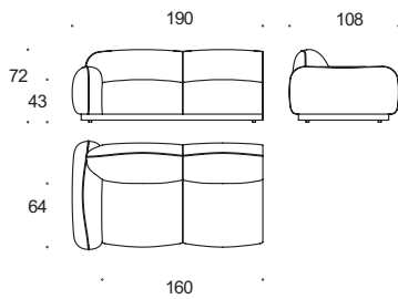
angolare corner element
