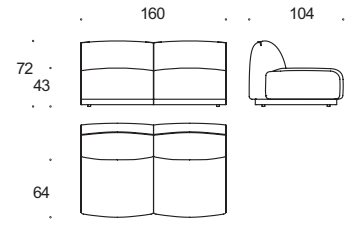
terminale 1P dx rh 1S end element
