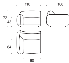
terminale 3P sx lh 3S end element
