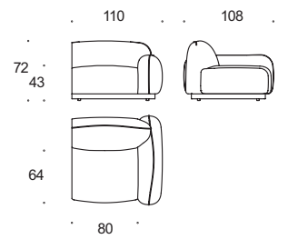
terminale 3P dx rh 3S end element
