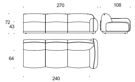
chaise longue sx lh chaise longue
